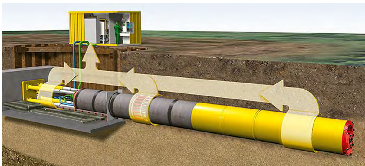
Figura 4: Esquema metodología constructiva pipe – jacking
