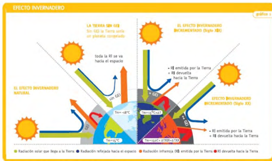
Figura 19: Diferentes escenarios posibles del efecto invernadero
